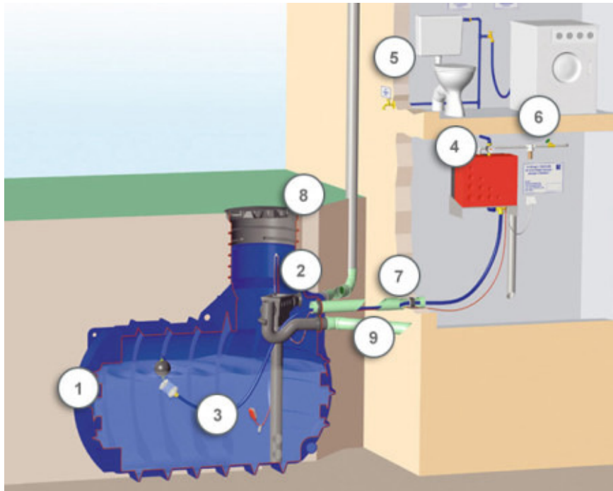
1-podzemni rezervoar BlueLine, 2-fini filter, 3-Črpalni set, 4-centralni krmilni sistem za deževnico, 5- varnostni paket, 6- filter za pitno vodo, 7- priključni kabel, 8-PE pokrov rezervoarja, 9- dotok
