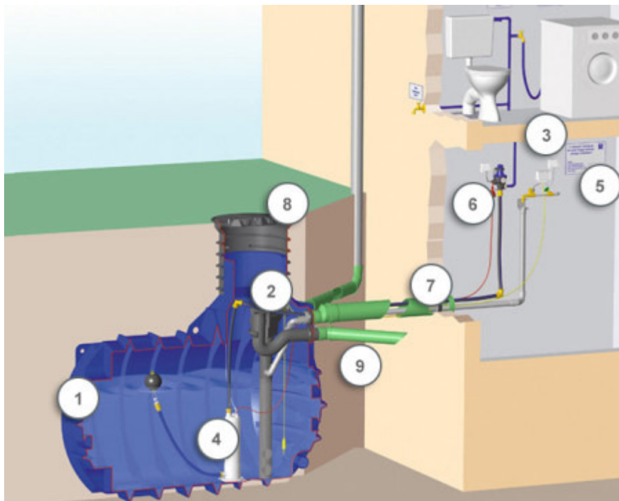
1-filtrirni rezervoar BlueLine, 2- fini filter, 3- dodatni priklop pitne vode, 4-potopna tlačna črpalka, 5-varnostni paket, 6- tlačno stikalo, 7- priključni kabel, 8-PE pokrov rezervoarja, 9- dotok
