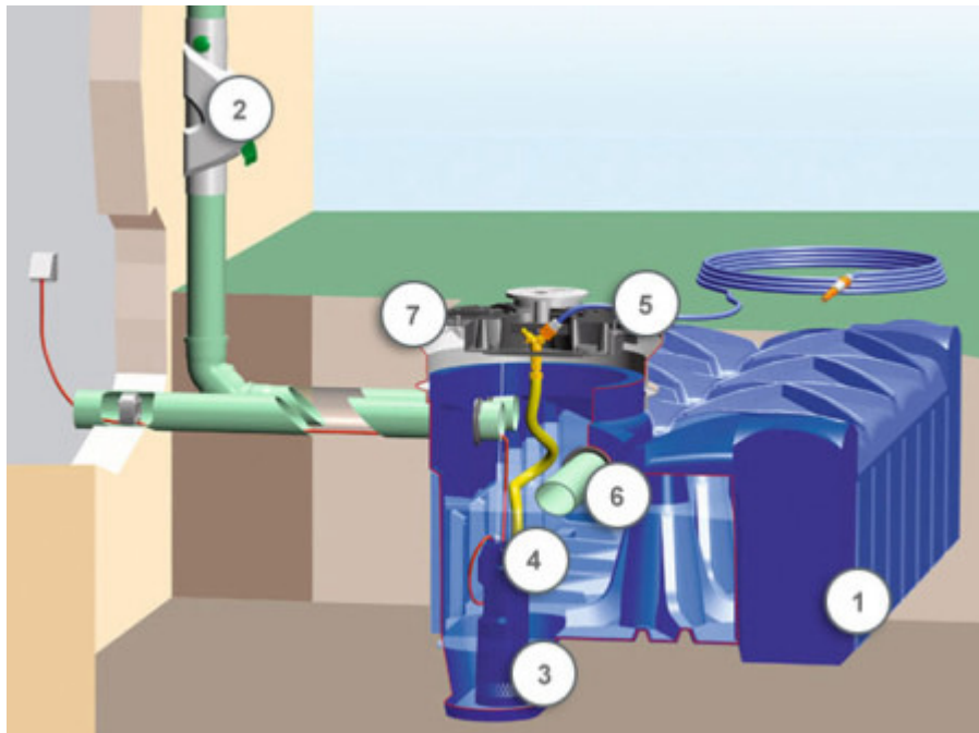
1-podzemni rezervoar F-LINE, 2-filter za žleb, 3-tlačna potopna črpalka, 4-tlačna cev, 5- pokrov rezervoarja z vgrajenim vodnim priključkom, 6-dotok, 7- podaljšek jaška
