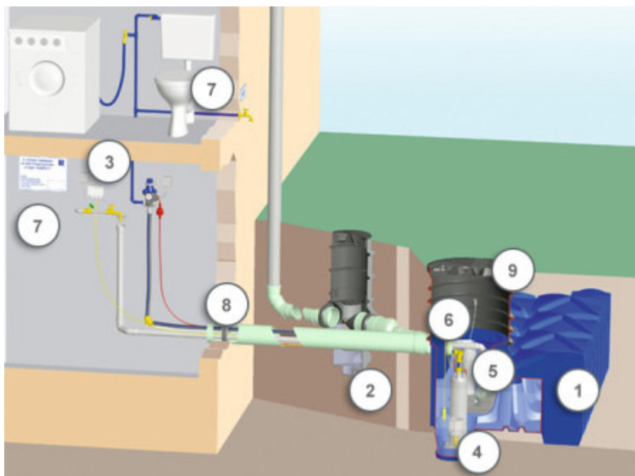
1-podzemni rezervoar F-LINE, 2-zunanji pred filter, 3- avtomatični priklop pitne vode, 4-potopna tlačna črpalka, 5-sifon za pretok rezervoarja, 6-kontrola pritoka, 7-varnostni paket, 8- priključni kabel, 9-PE pokrov rezervoarja
