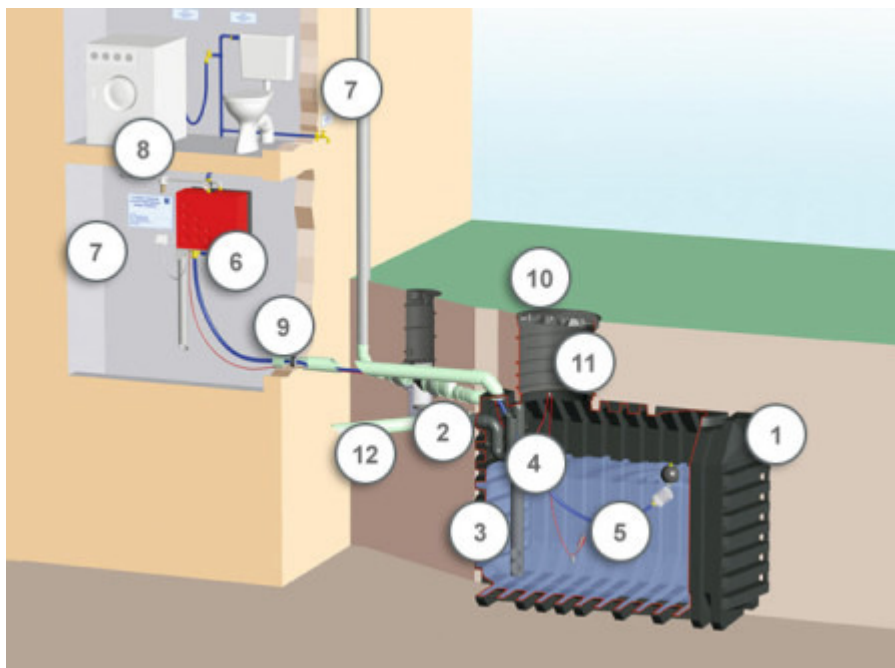
1-Rezervoar MONOLITH, 2-predfilter, 3- kontrola dotoka, 4- sifon za pretok, 5- črpalni set s finim filtrom, 6- centralni krmilni sistem za deževnico, 7-varnostni paket, 8- - filter za pitno vodo, 9- - priključni kabel, 10- PE pokrov rezervoarja, 11- podaljšek jaška, 12- dotok
